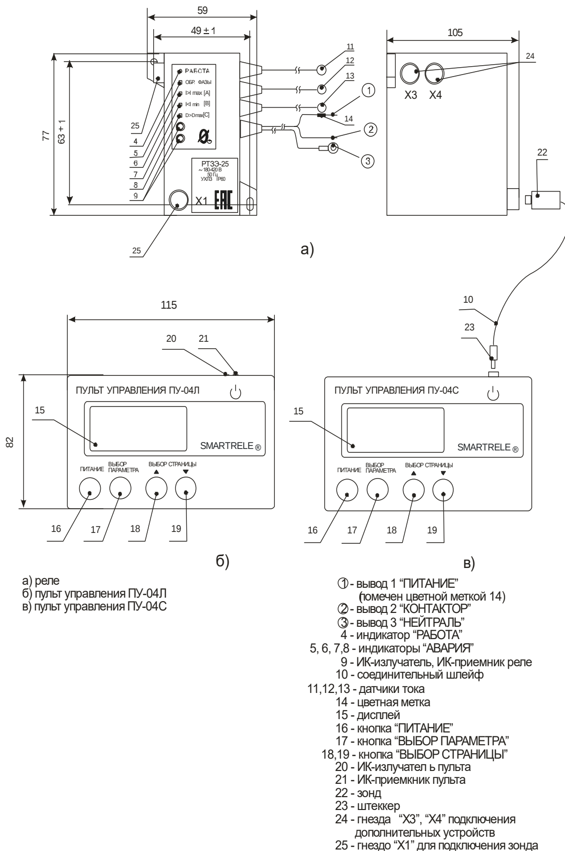
Рисунок 1 – общий вид реле модификаций РТЗЭ, РТЗЭ-С и пультов, расположение их органов индикации и управления
